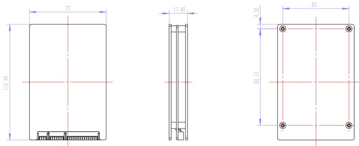
JK-BD4A17S/20S-4P 外形尺寸
