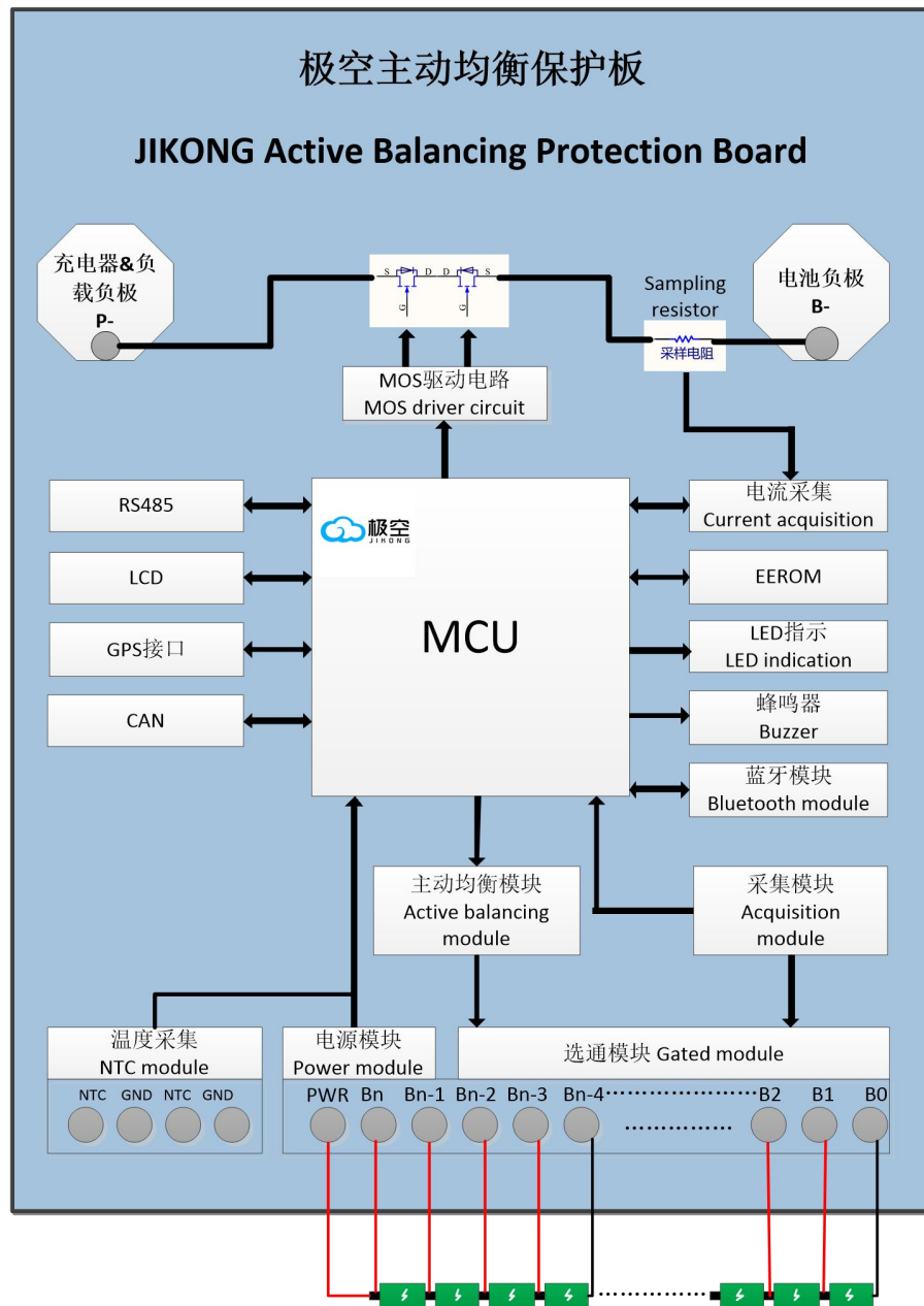
JK-BD4A24S-4P 结构框图
