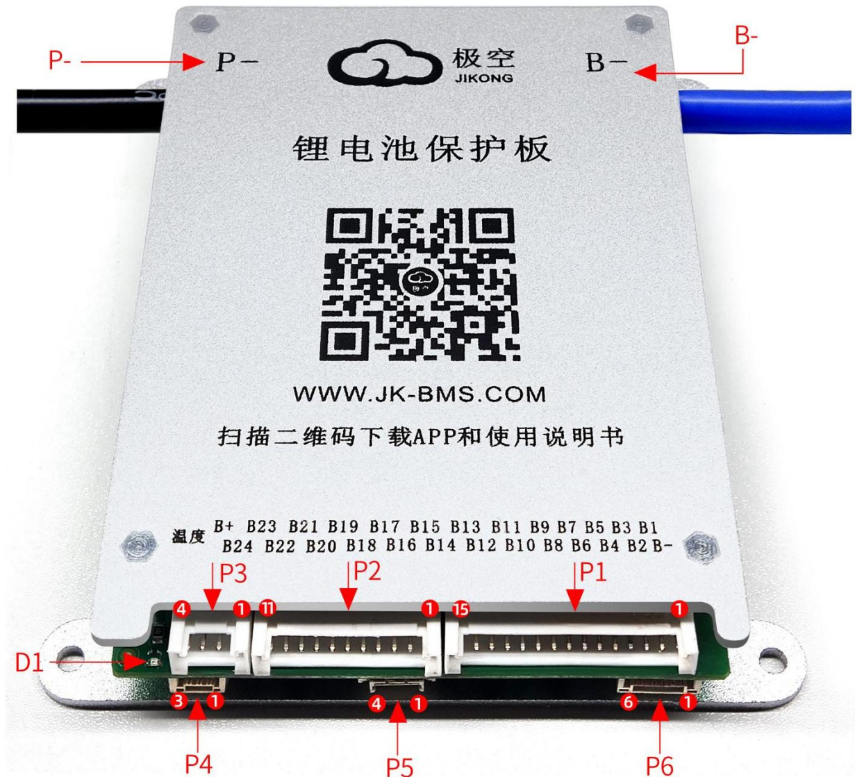
JK-BD4A24S-4P 连接器示意图
