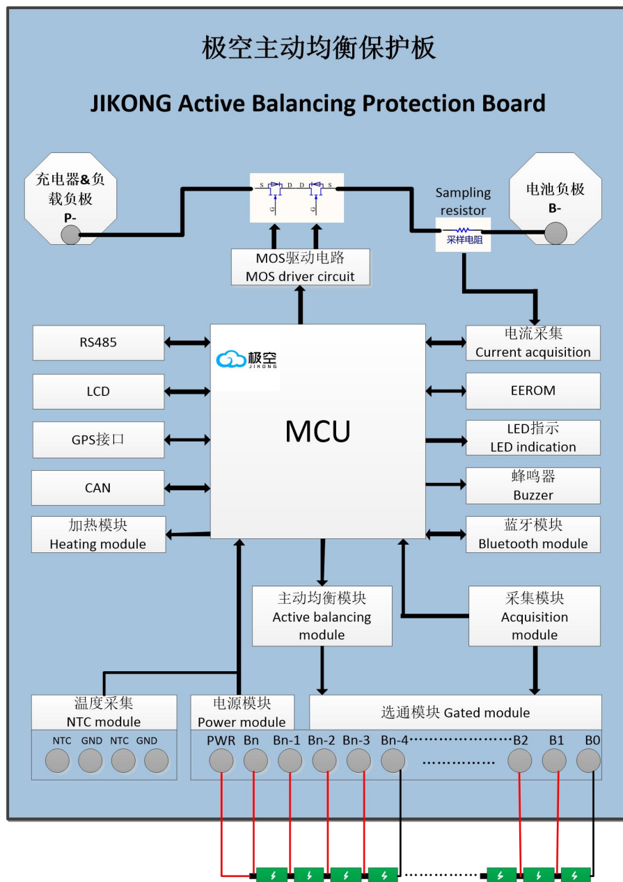
JK-BD6A20/24S-12P 结构框图
