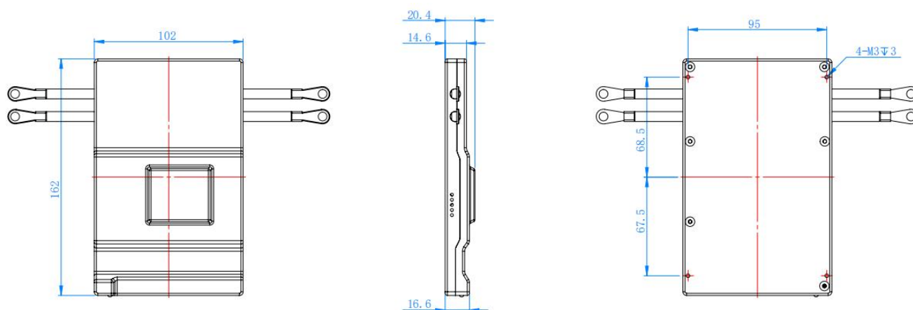
JK-BD6A20/24S-12P 外形尺寸
