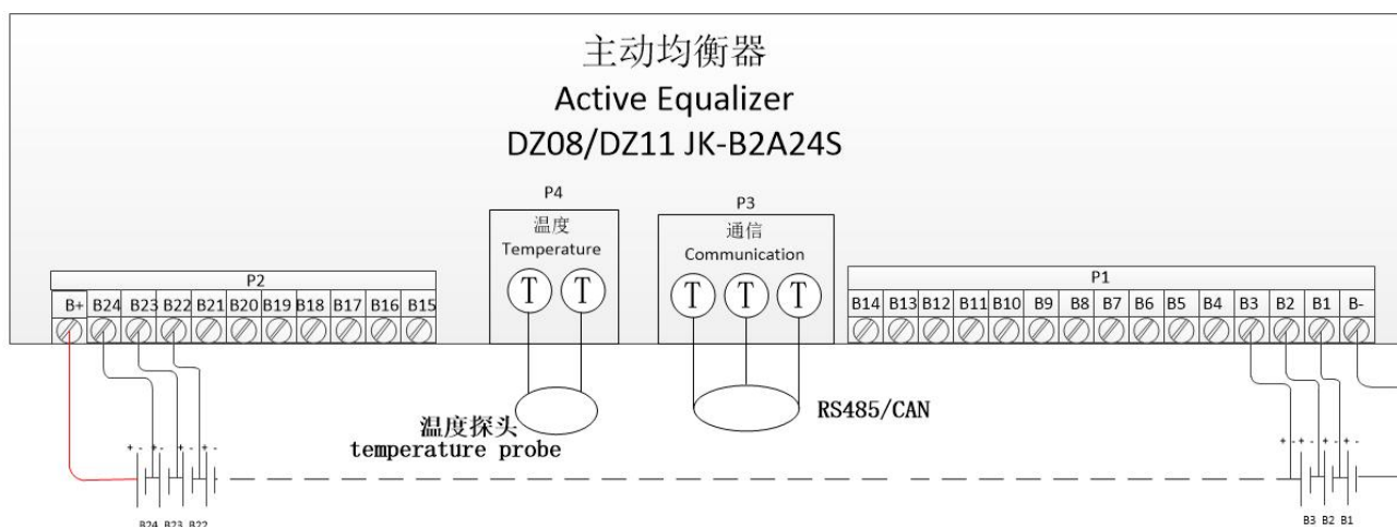
JK-B2A24S 接线图
