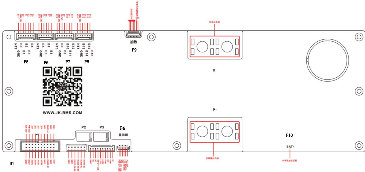
JK-PB1/2A16S-10/15/20P 连接器示意图
