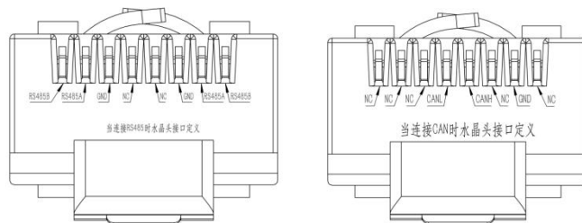
接口板接口示意图
