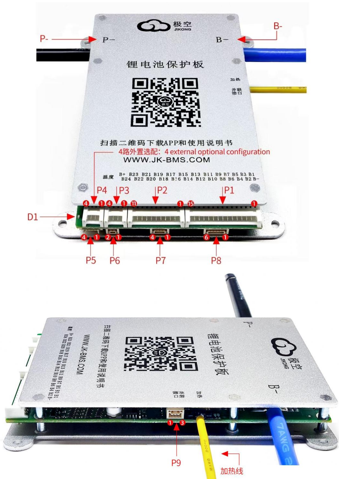
JK-BD6AxxS-6P/8P连接器示意图
