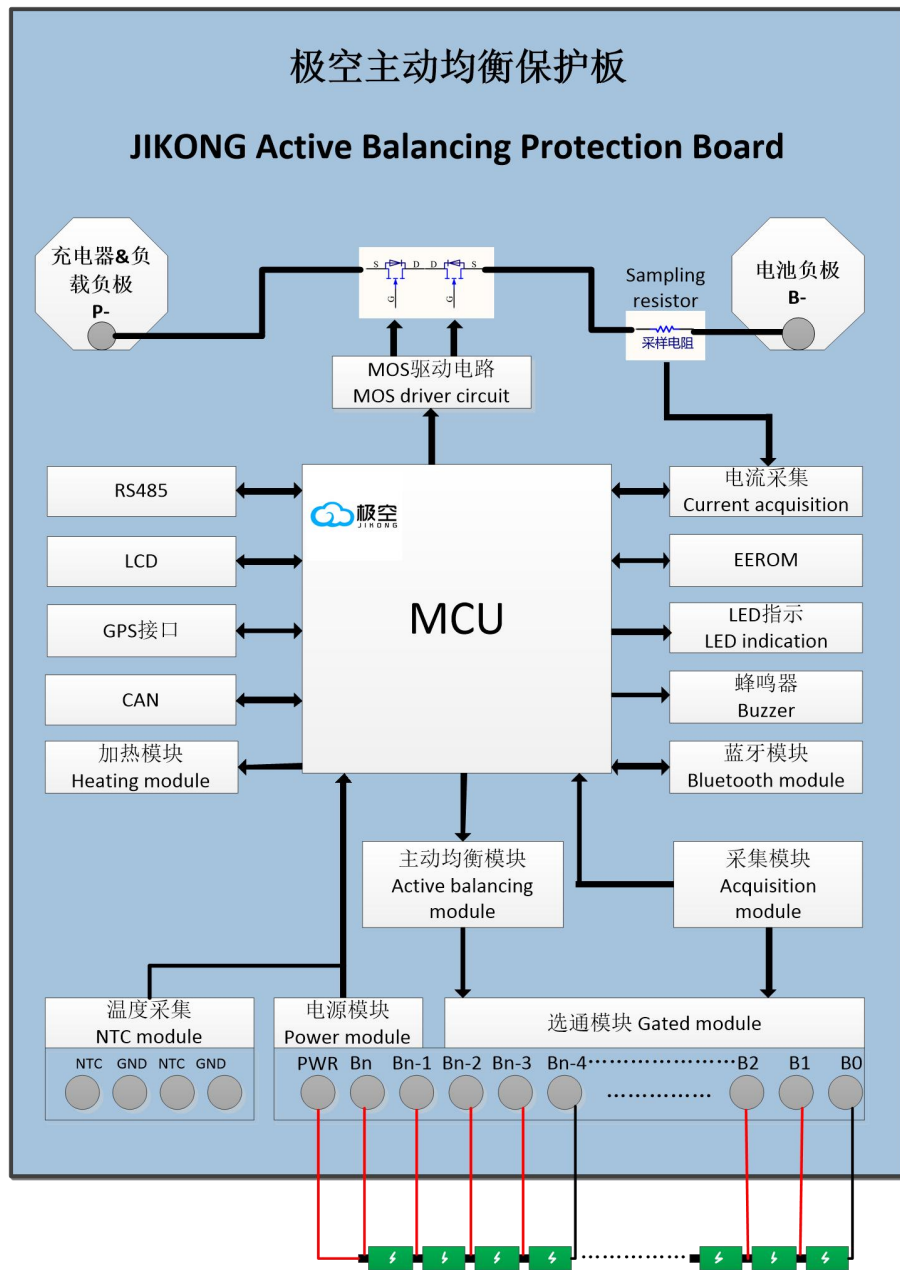
JK-BD6A20/24S-15P-20P结构框图
