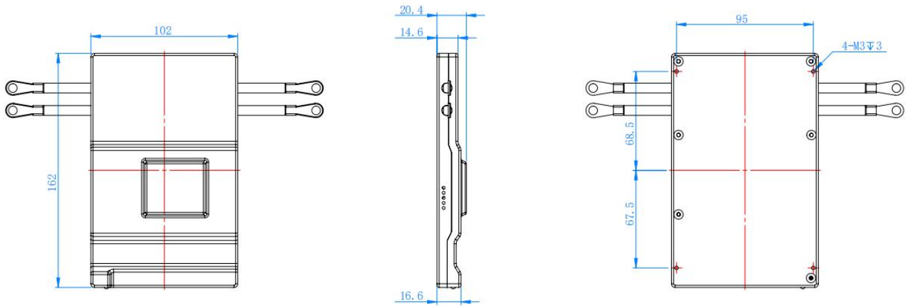
JK-BD6AxxS-15P/20P 外形尺寸
